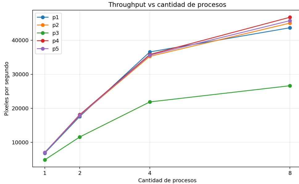
Figura 4: Throughput según la cantidad de procesos.
